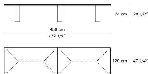
tavolo conferenza rettangolare rectangular conference table
