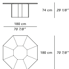
tavolo conferenza ottagonale octagonal conference table
