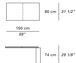
sezione centrale tavolo conferenza conference table, central unit
