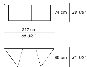
sezione frontale tavolo conferenza conference table, terminal unit
